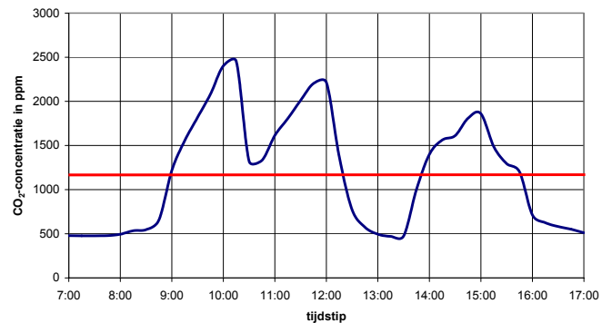
kenmerkend verloop CO 2 concentratie in leslokaal
